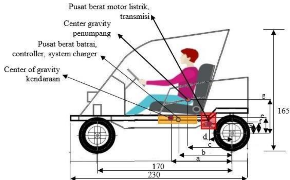
Gambar Rencana desain kendaraan dan titik berat
