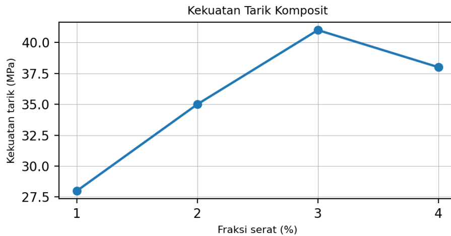
Gambar 1. Pengaruh Fraksi Serat Bambu terhadap Kekuatan Tarik
