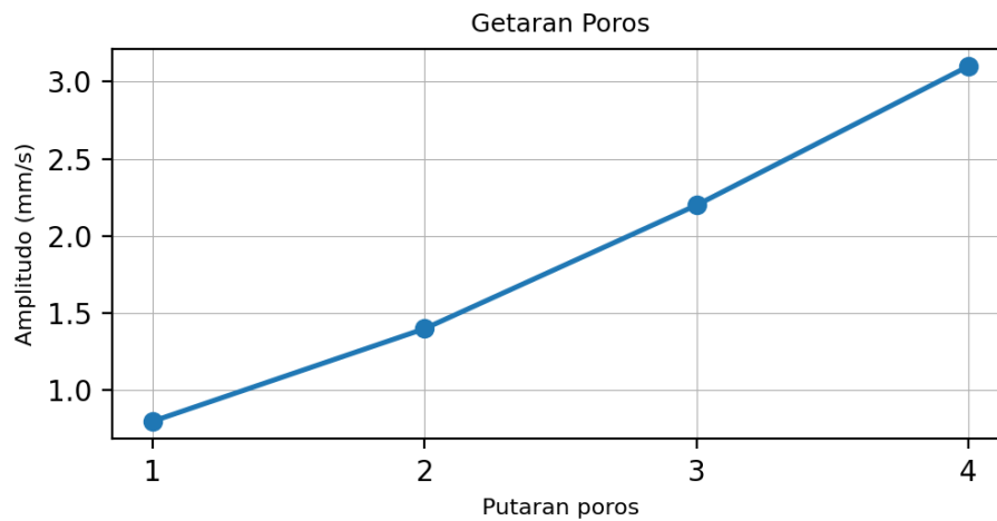
Gambar 1. Hubungan Putaran Poros dan Amplitudo Getaran
