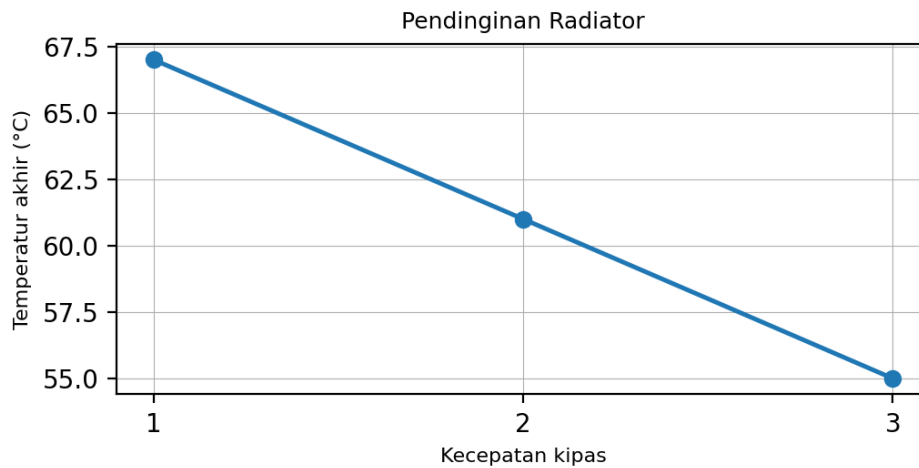
Gambar 1. Pengaruh Kecepatan Kipas terhadap Temperatur Akhir
