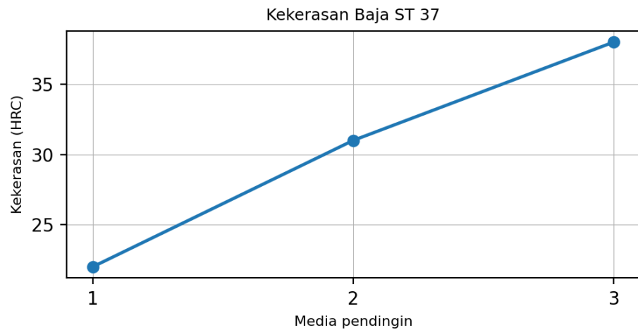
Gambar 1. Pengaruh Media Quenching terhadap Kekerasan Baja ST 37
